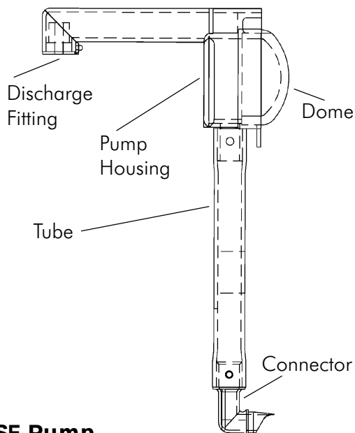
SE Pump
